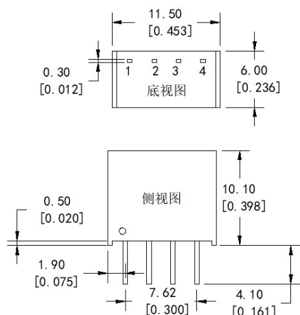
封装尺寸图
